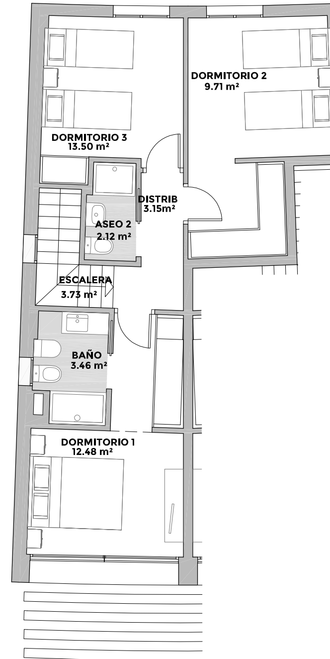
PLANTA PRIMERA
