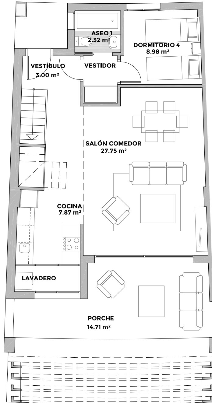
PLANTA BAJA
